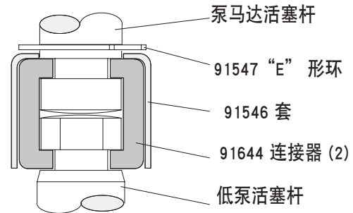
泵连接详图
