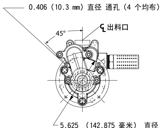
底视图
