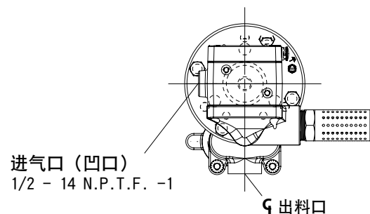
顶视图
